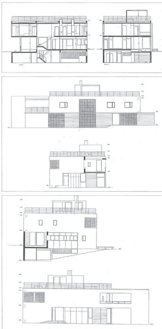
Casa riangolare a Espluges de Llobregat (Barcellona). Prospetti e sezioni.
